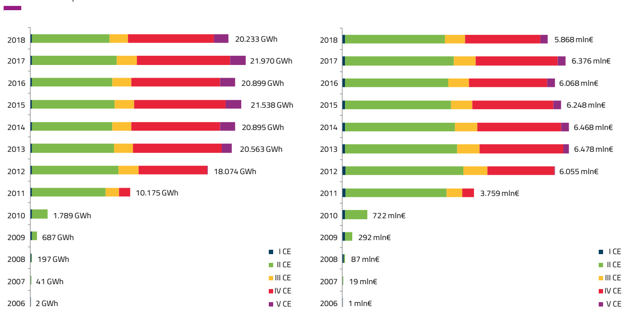
FIGURA 29 - Evoluzione dell'energia incentivata (a sinistra) e dei corrispettivi erogati (a destra) agli impianti fotovoltaici per CE di riferimento
