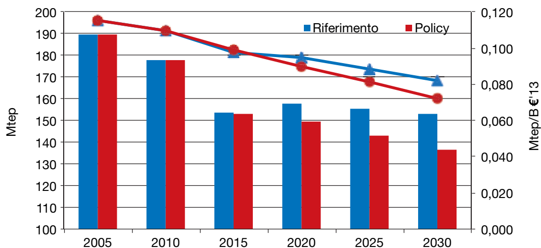
Figura 39: Evoluzione del fabbisogno primario di energia e dell'intensità energetica [Fonte: Elaborazione ENEA]
