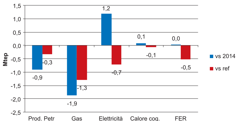
Figura 45: Variazione dei consumi per fonte nel settore terziario nel 2030 rispetto al 2014 e rispetto al Riferimento [Fonte: Elaborazione ENEA]
